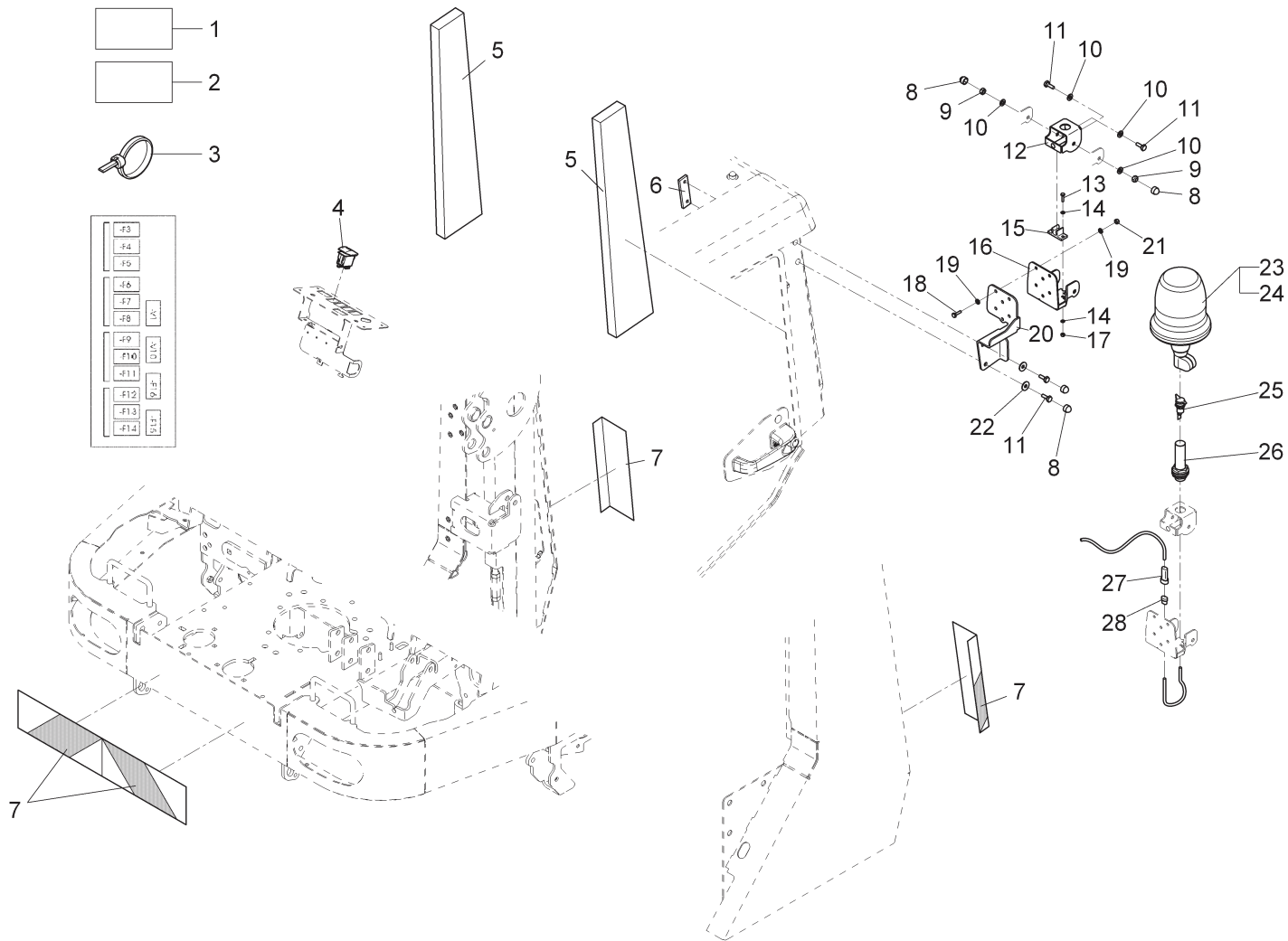
Abb.1 Zusammenbau
